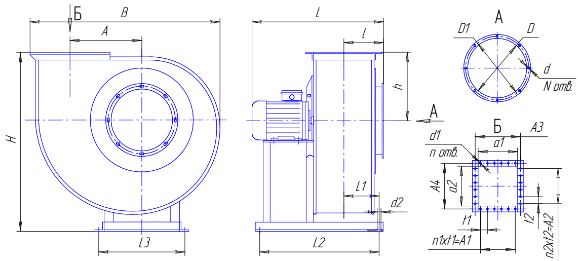
Исполнение 5-01
