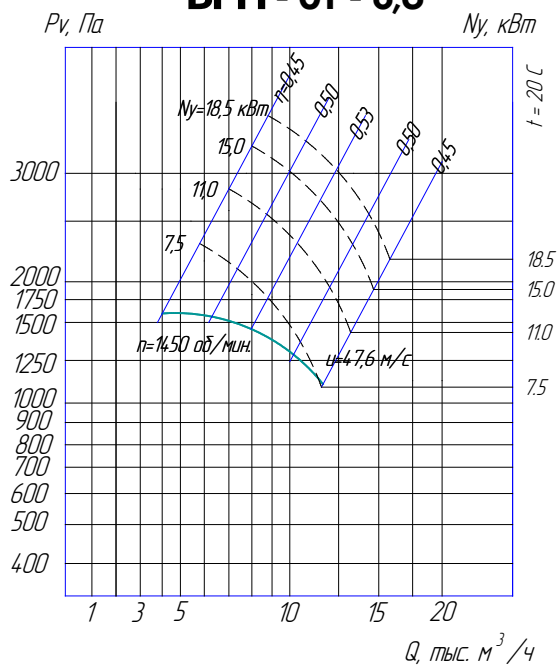
ВРП - 01 - 6,3
