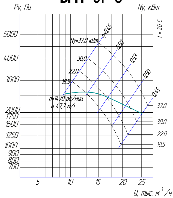
ВРП - 01 - 8
