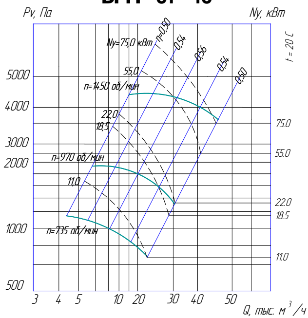
ВРП - 01 - 10
