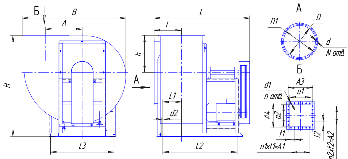
Исполнение 5-02
